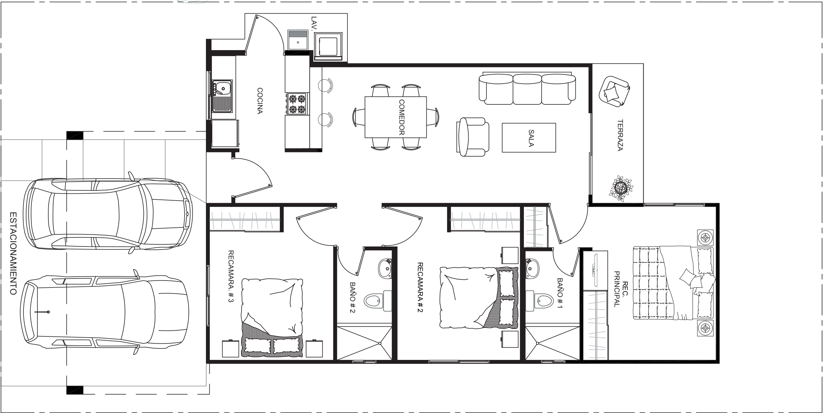
PLANTA ARQUITECTONICA CASA VILLAS DEL NORTE PROPUESTA MACRO
